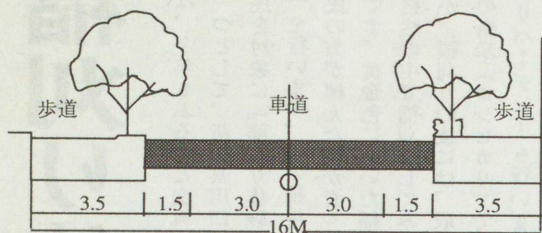
都市計画道路（16Mの幅員の場合）標準断面図
