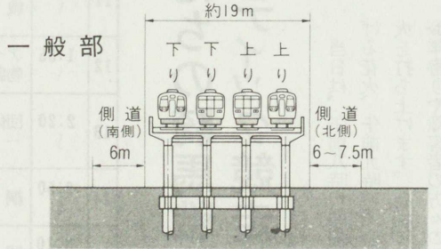
小田急線立体化と環境側道整備横断面図
