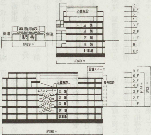
再開発ビル断面概要図
