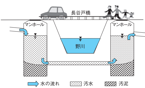
伏越しのしくみ
